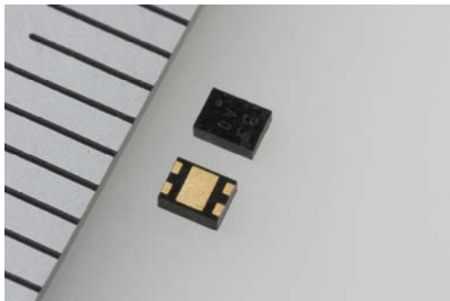
▲XC6503 シリーズ、USP-4 (1.2 x 1.6 x h0.6mm)
