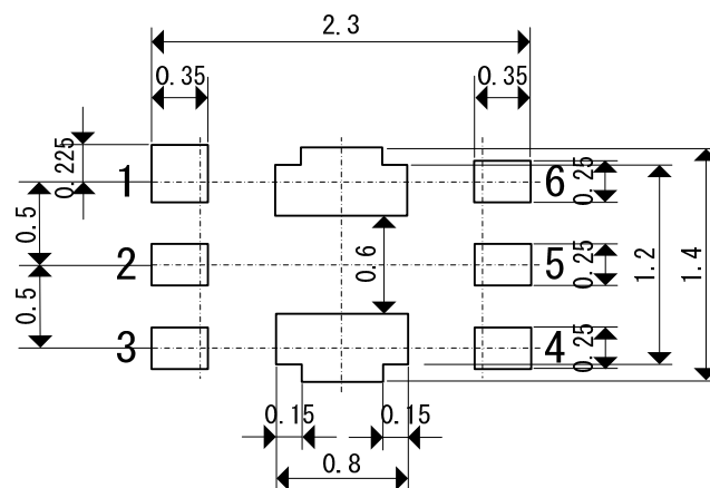
●USP-6C 参考メタルマスクデザイン
