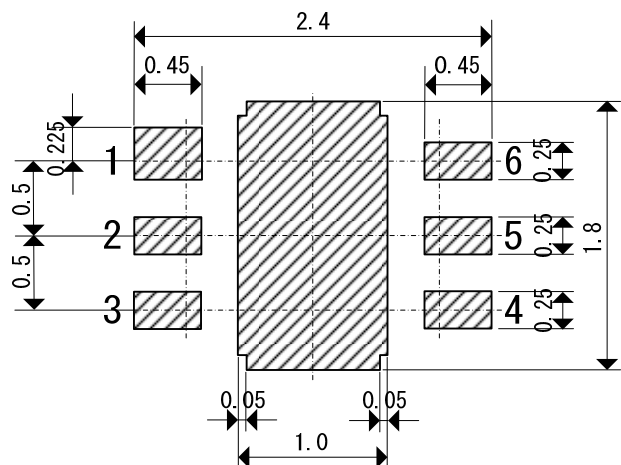
●USP-6C 参考パターンレイアウト
