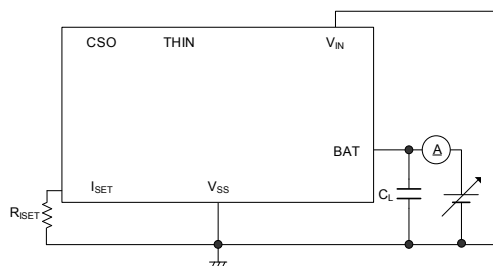
6) 測定回路⑥
