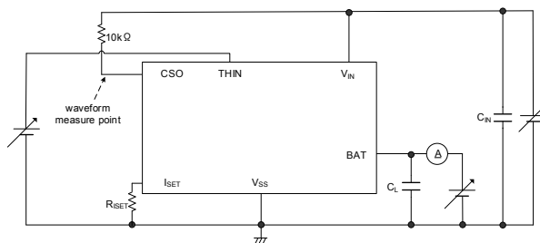
4) 測定回路④
