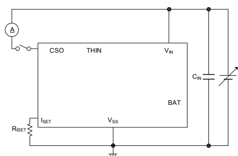
7) 測定回路⑦
