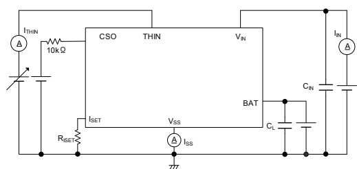
3) 測定回路③
