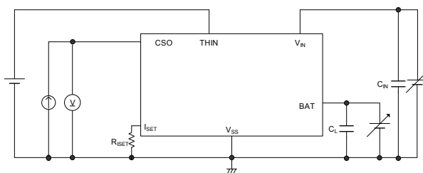
6) 測定回路⑥
