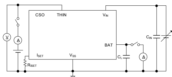
7) 測定回路⑦
