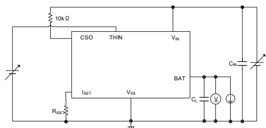
5) 測定回路⑤
