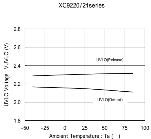
UVLO温度特性例
