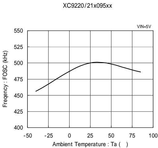
発振周波数温度特性例
