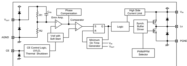
3) XC9260/XC9261 シリーズ A タイプ(USP-6C)
