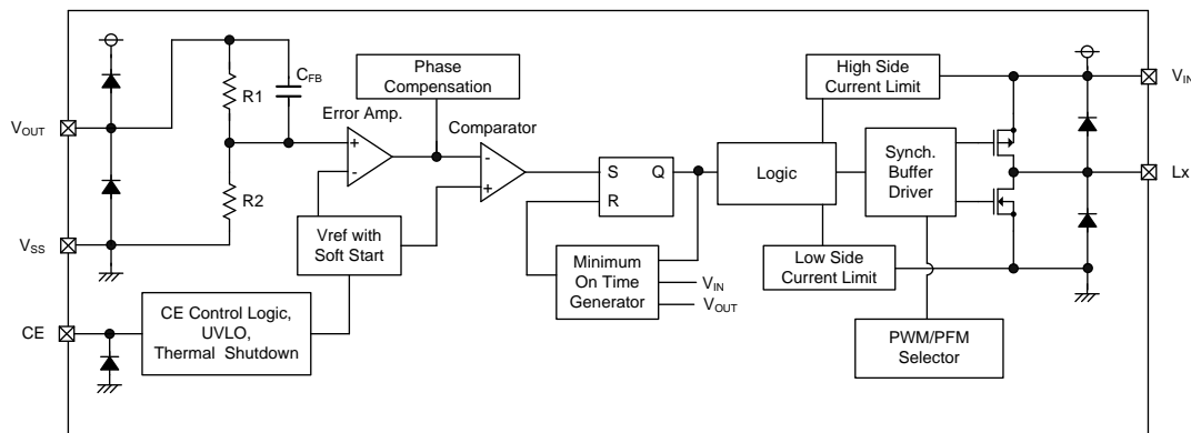
BLOCK DIAGRAM (XC9260/XC9261 シリーズ B タイプ(SOT-89-5))
