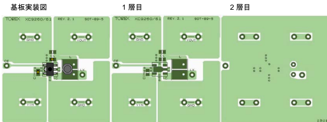
USP-6C 基板実装図
