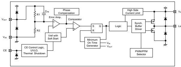
1) XC9260/XC9261 シリーズ A タイプ(SOT-89-5)
