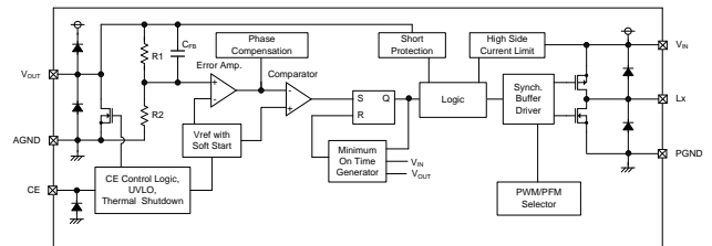
4) XC9260/XC9261 シリーズ B タイプ(USP-6C)
