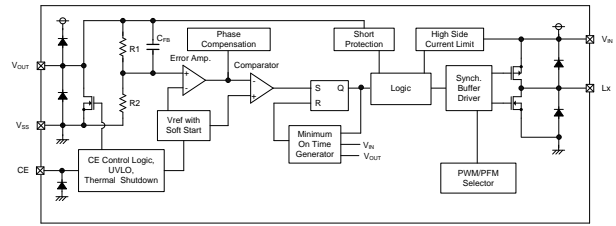
2) XC9260/XC9261 シリーズ B タイプ(SOT-89-5)
