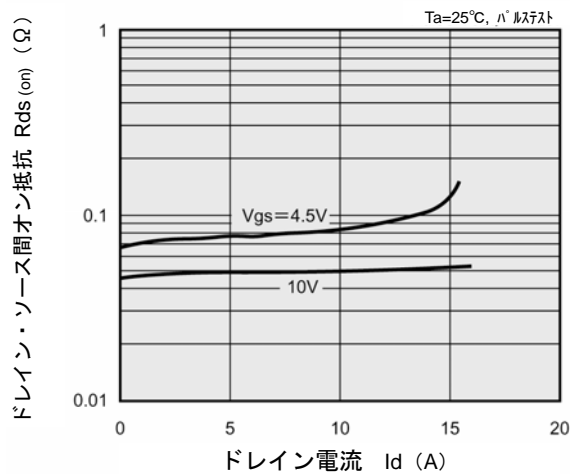
(4) ドレイン・ソース間オン抵抗-ドレイン電流 特性例
