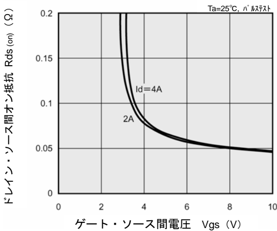
(3) ドレイン・ソース間オン抵抗-ゲート・ソース間電圧 特性例
