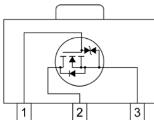
Nチャンネル MOSFET (1素子内蔵)
