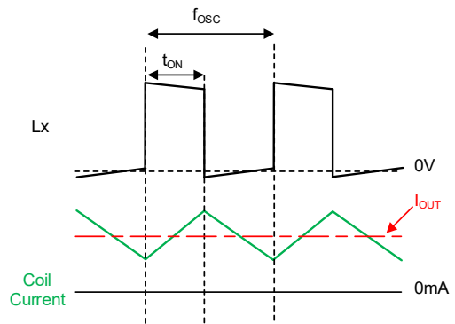
XCL239 シリーズ : 重負荷動作例
