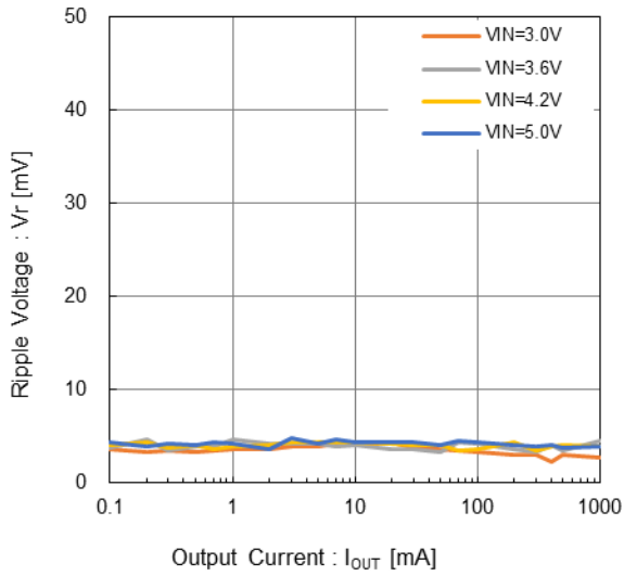
XCL239 V_{OUT(T)}=1.8V
