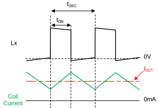
XCL240 シリーズ : 重負荷動作例
