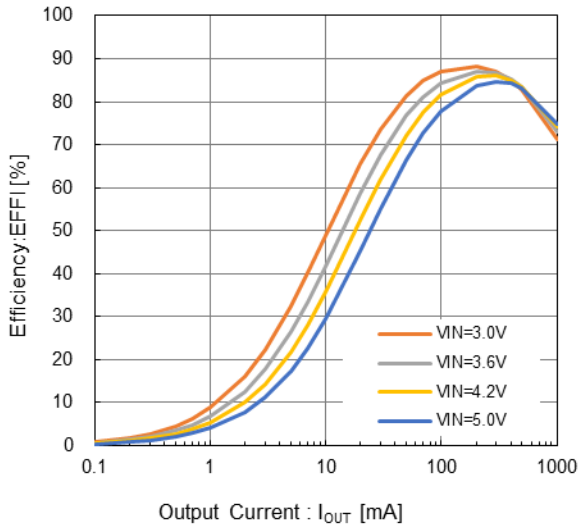
XCL239 V_{OUT(T)}=1.8V
