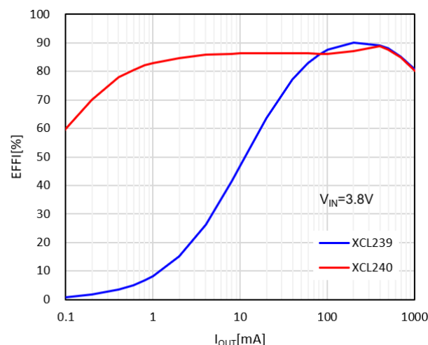
XCL239/XCL240 (V OUT =1.8V)
